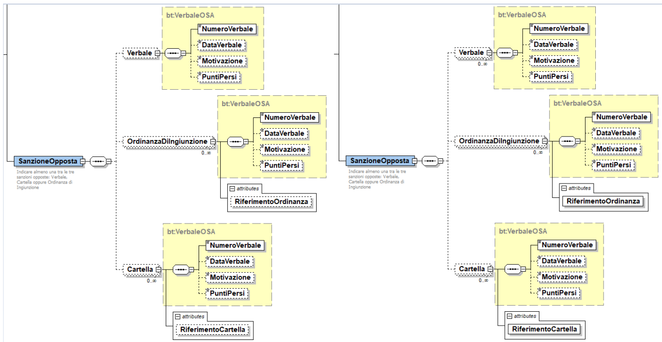
Figura 1 - Nuovo XSD per OSA
