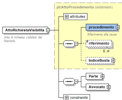
Figura 3 - AttoRichiestaVisibilita
