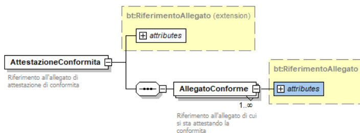
Figura 2 - AttestazioneConformita
